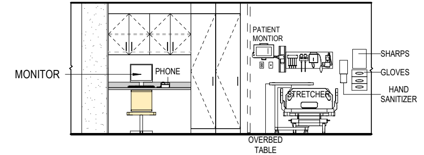
ELEVATION 01
